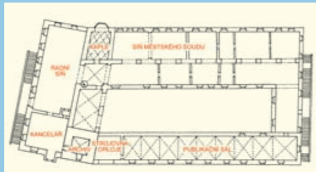
Оломоуцкая ратуша в конце 16 века. План первого этажа.
